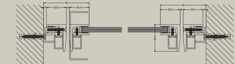
PORTE PIVOTANTE
