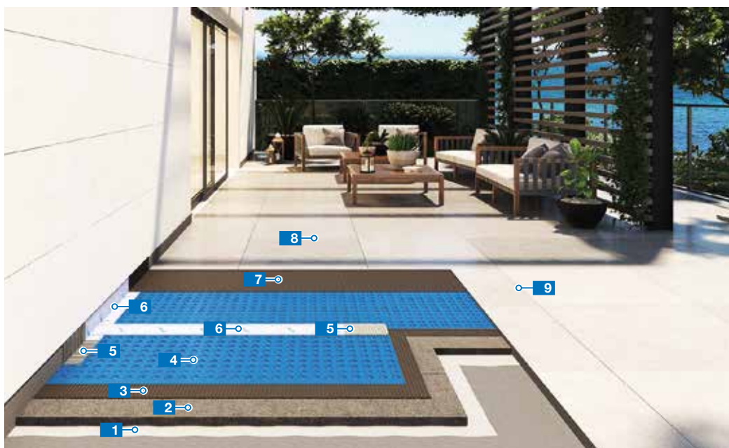
Imperméabilisation des contours avec Mapeband Easy, collée avec Mapeguard WP Adhesive
